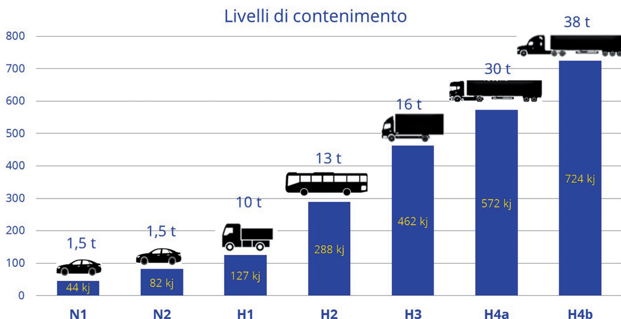
Figura 4-3: Livelli di contenimento e mezzi impiegati nelle diverse prove
