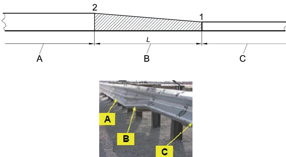
Figura 8-14: Identificazione degli elementi di una transizione
