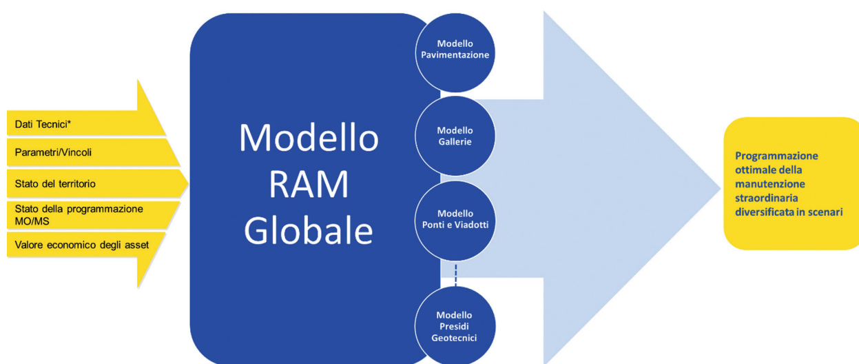
Figura 2-1: Schema logico del modello RAM
