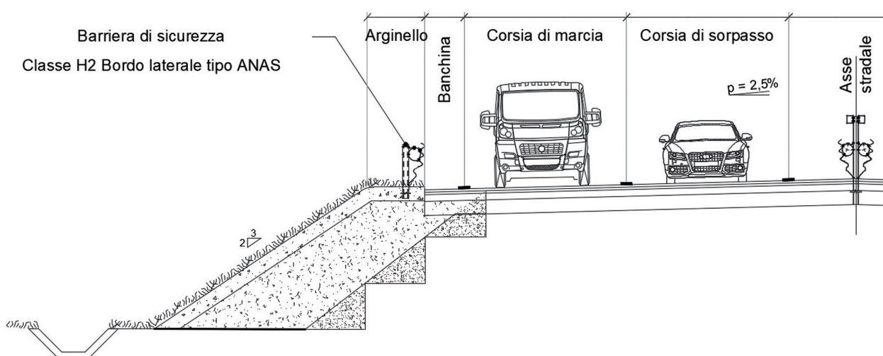
Figura 5-4: Supporto tipo reale del bordo laterale
