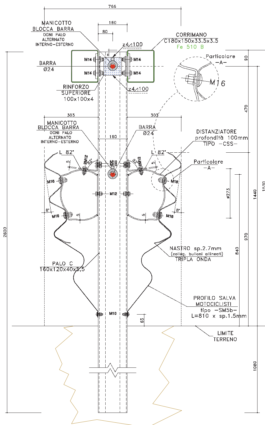
BARRIERA ANAS H4ST DSM Monofilare (interasse 1500mm) ELEMENTO ASSEMBLATO SCALA 1:10
