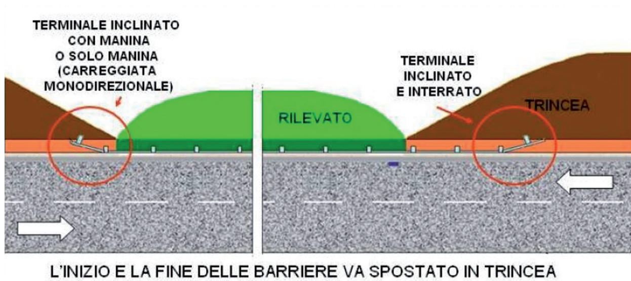
Figura 8-4: Posizionamento del terminale semplice
