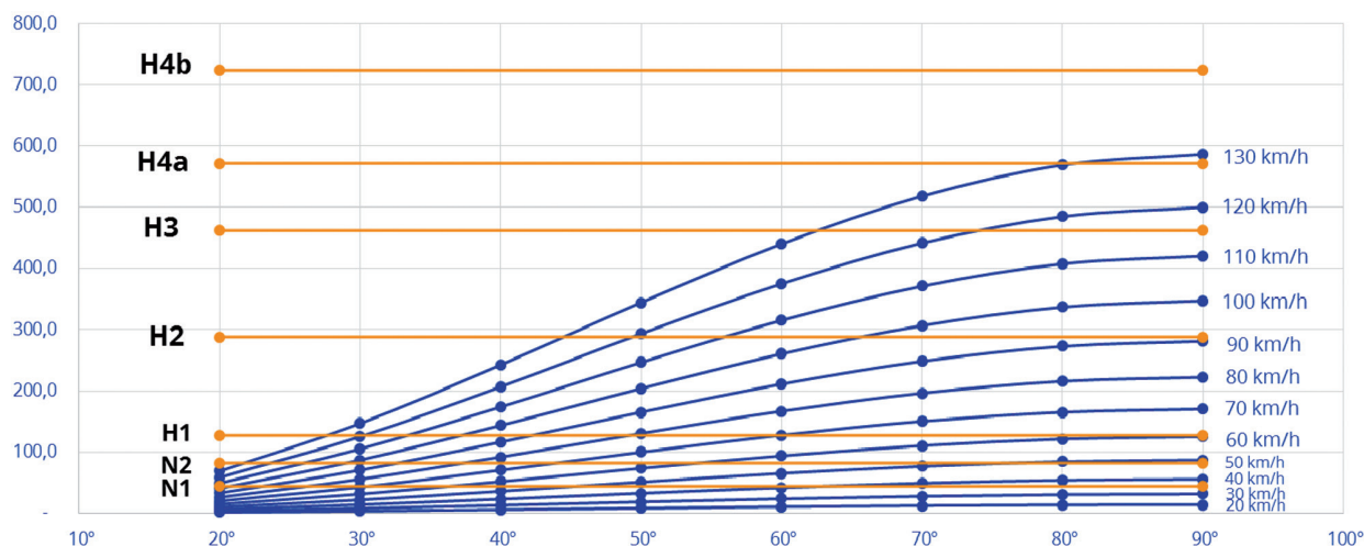
Figura 4-4: L_c [kJ] al variare di V [km/h] e \theta [°]
