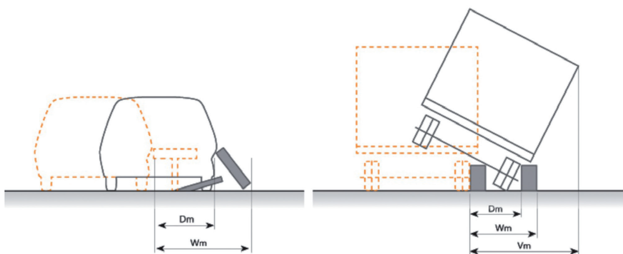
Figura 4-9: Schemi per la misura dei parametri geometrici D_m , W_m , V_m
