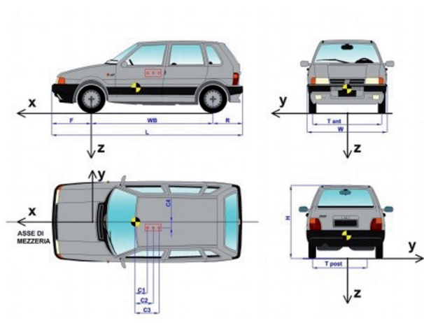
Figura 4-7: Dimensioni del veicolo (prova TB11)
