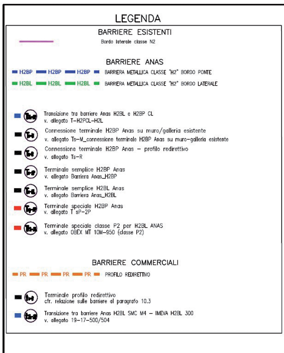
Figura 5-3: Legenda schema di intervento
