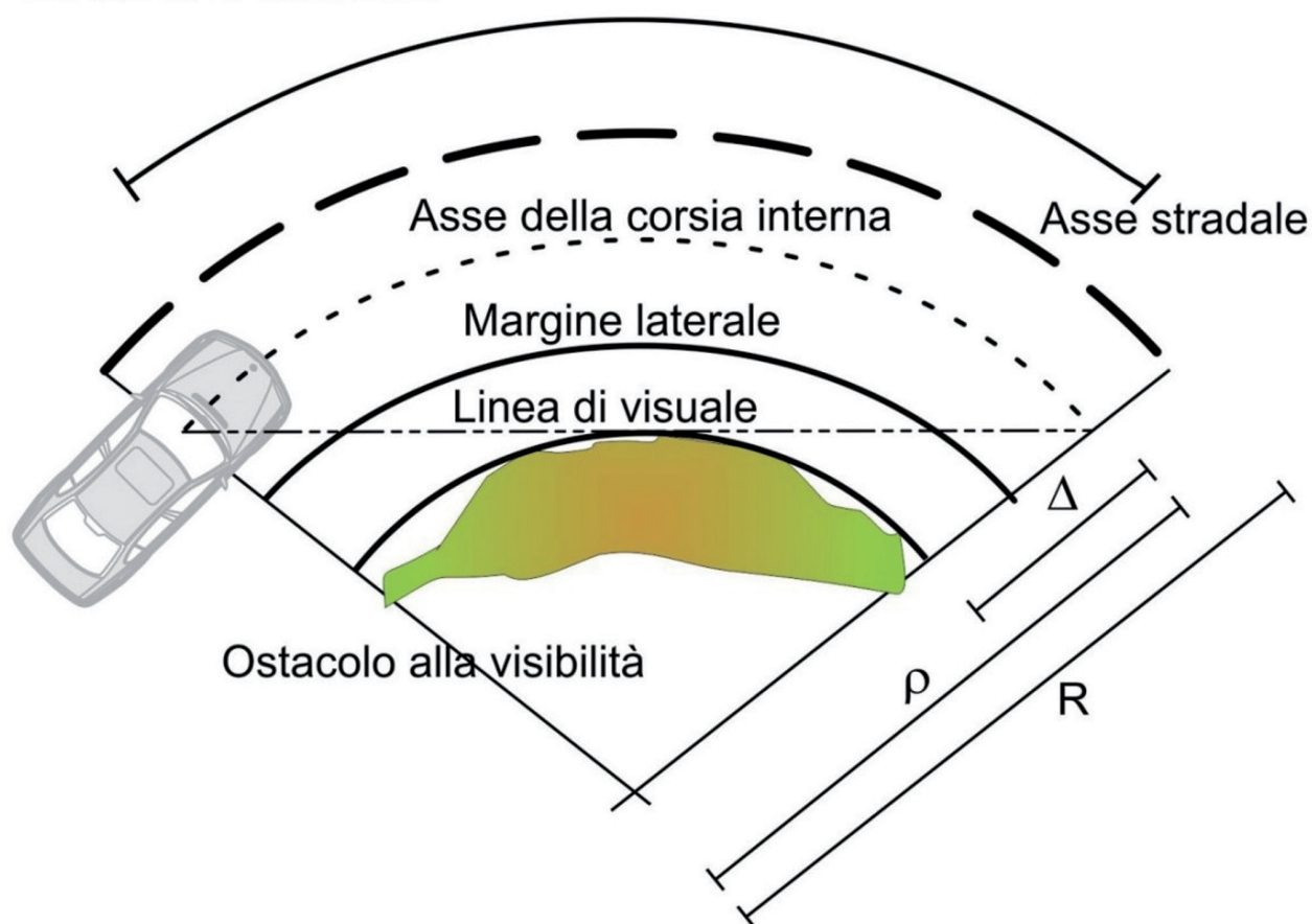
Figura 6-1: Schema di controllo della visibilità in curva
