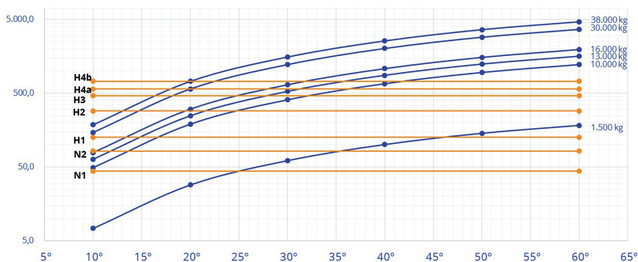
Figura 4-5: Andamento di L_c [kJ] al variare di M [kg] e \theta [°]
