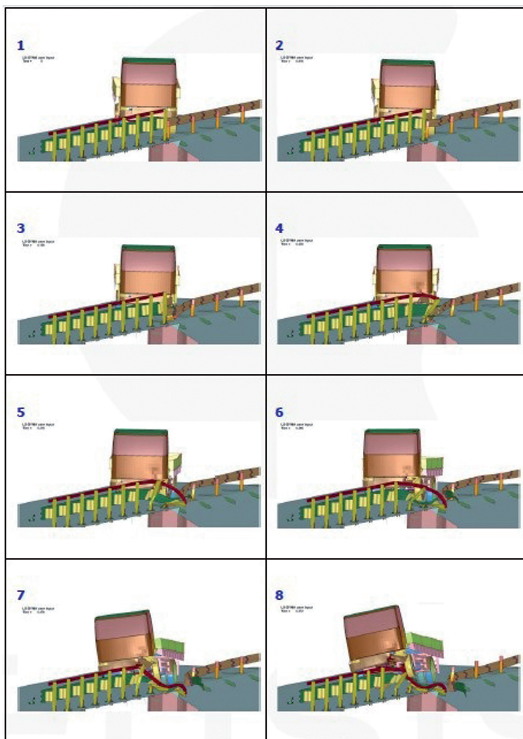
Figura 8-19: Verifica del comportamento della transizione [13]
