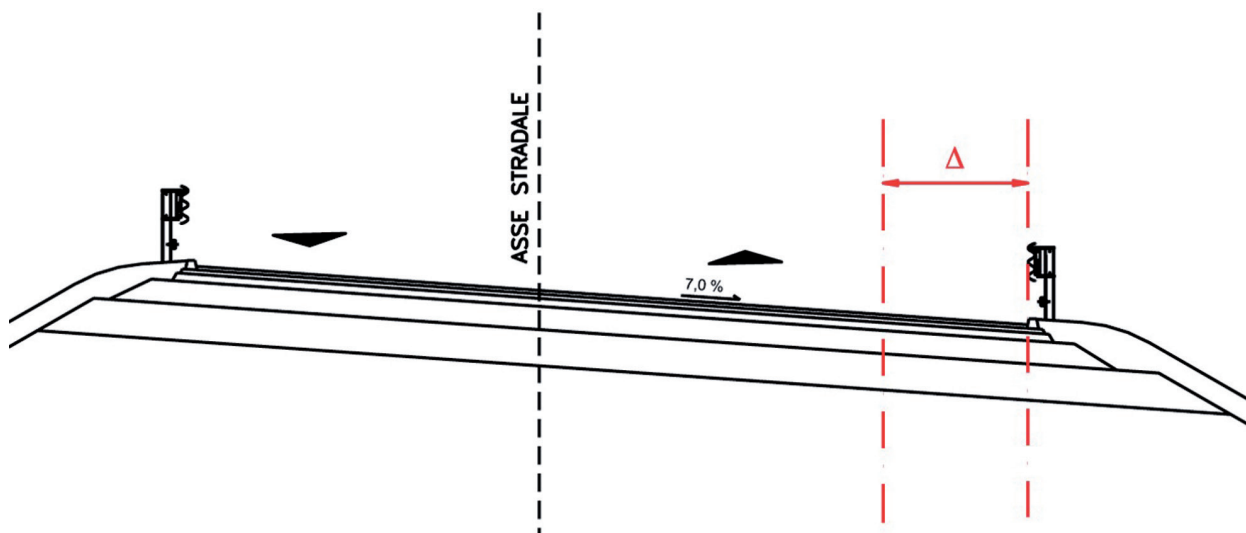
Figura 6-2: Schema di allargamento della banchina
