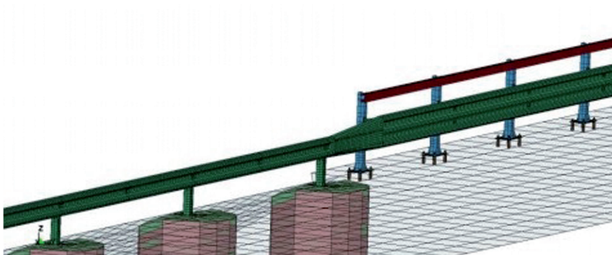
Figura 8-17: Transizione da verificare [13]
